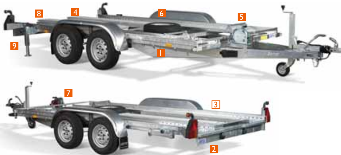
4 Sicherungsverschluss
